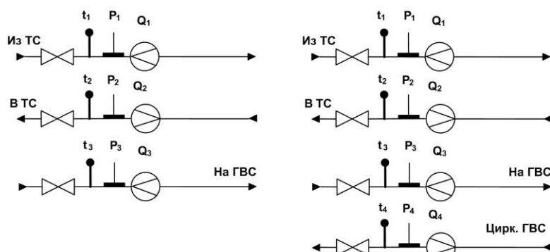
Рис.4. Схемы теплоснабжения с подпиткой из различных трубопроводов
