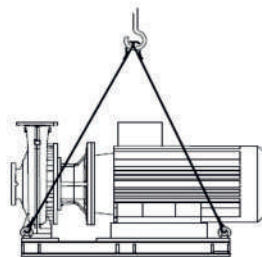
Рис. 2 Правильный способ строповки насоса с плитой-основанием
