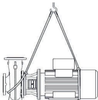
Рис. 1 Правильный способ строповки насоса без плиты-основания
