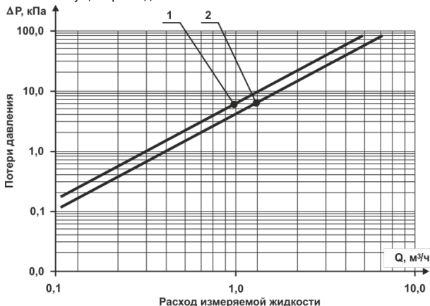
1 – КАРАТ-Компакт 2–223 (Ду15); 2 – КАРАТ-Компакт 2 – 223 (Ду20)
